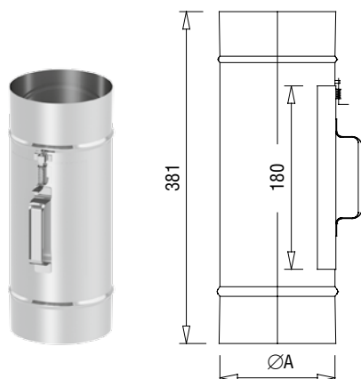
KL07 Ревизия с прямоугольным лючком до 400°C под разрезением
