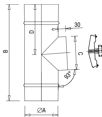
KL07r Ревизия-тройник до 400°C под разрезением
